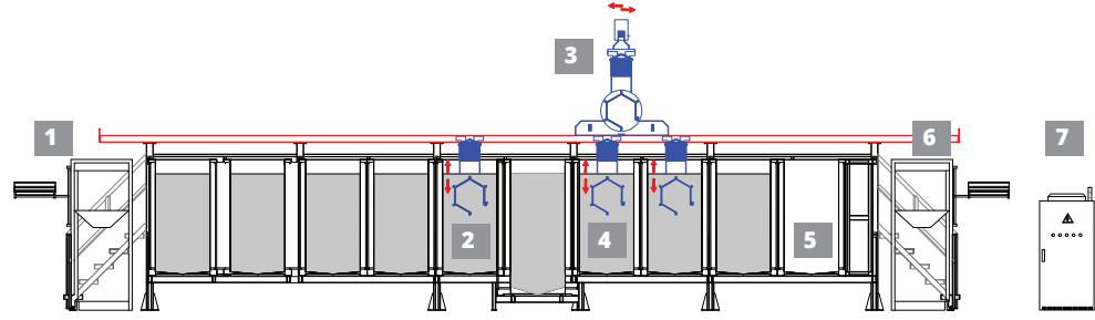
Gösterilen Model: Çinko fosfat hattı örneği Shown model: Zinc phosphate process example
